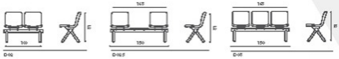
Teknik çizim
