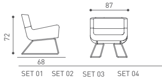
Teknik detay
